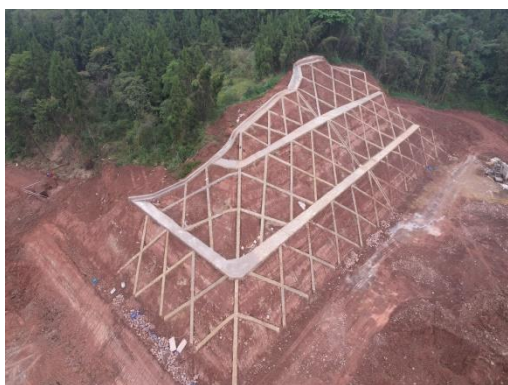
图3.1-3 浆砌片石骨架铺草皮护坡（骨架）
